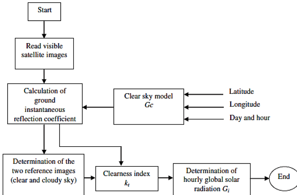
Fig. 15. GISTEL steps [245].
