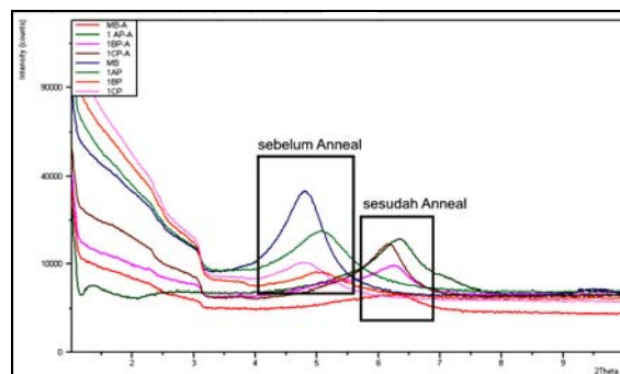
Gambar 5. Perbandingan hasil XRD sebelum dan sesudah anil
