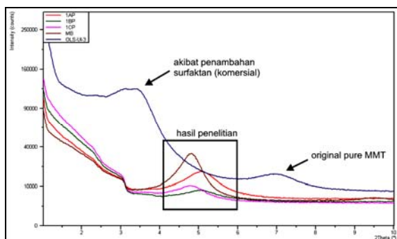
Gambar 3. Grafik perbandingan hasil XRD pure OLS tanpa OH - dengan 1AP, 1BP, 1CP, dan MB
