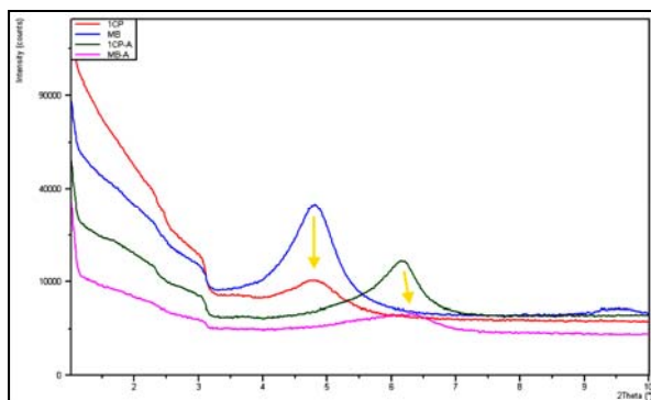
Gambar 4. Pola difraksi sinar-X sebelum dan sesudah annealing PPCN dan masterbatch dengan waktu proses 6 menit
